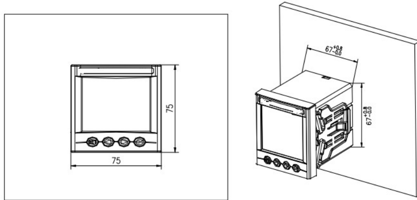
图 3 PM72B 安装尺寸
