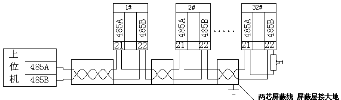
图 10 RS485 通讯接线示意图
