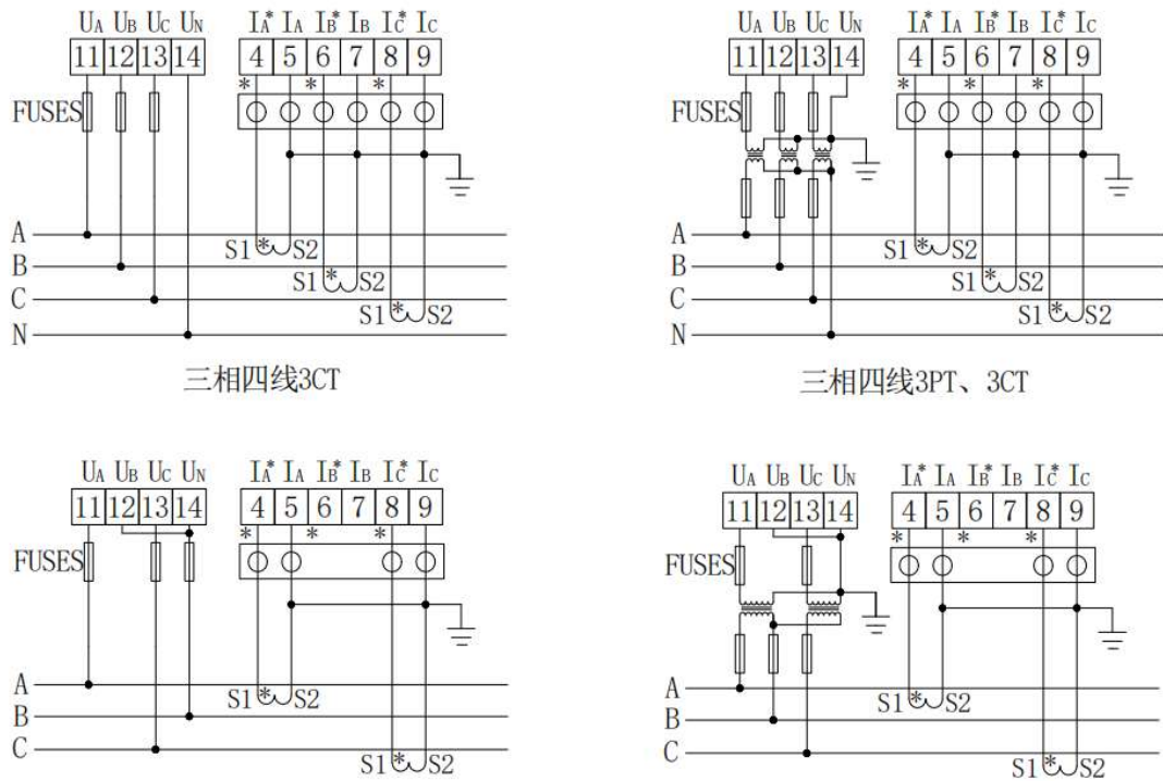
图 9 仪表信号接线示意图
