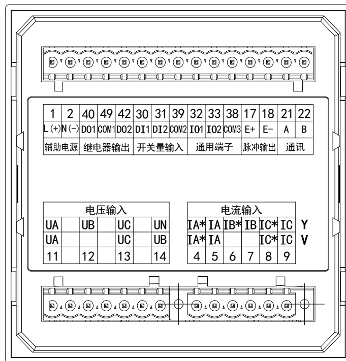
图 8 PM96B 系列接线端子图
