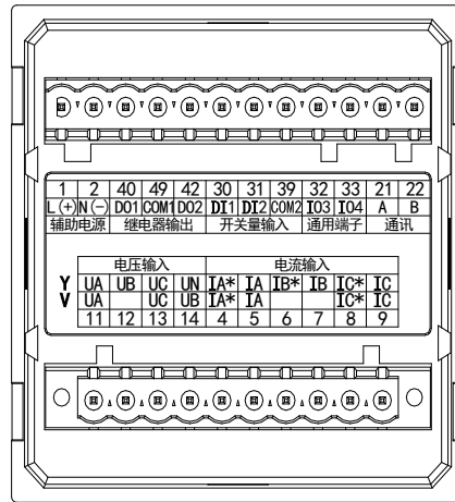
图 7 PM72B 系列接线端子图
