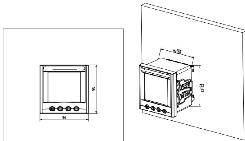
图 4 PM96B 安装尺寸
