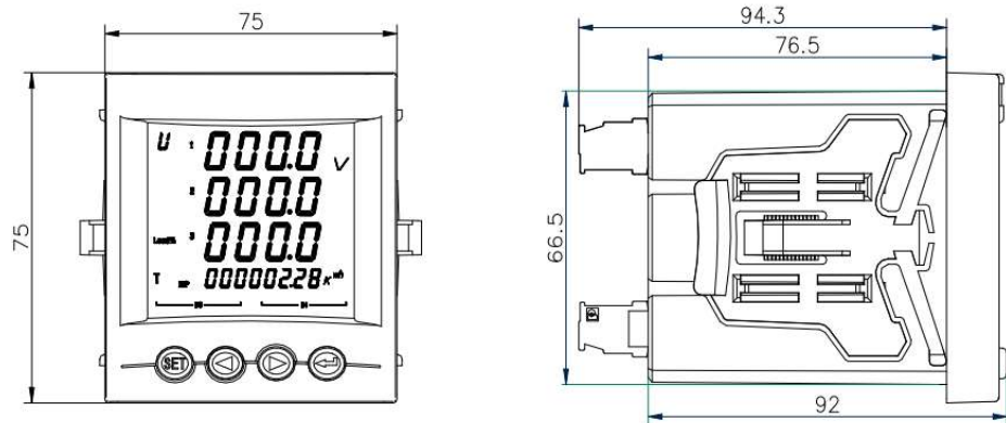
图 1 PM72B 外观尺寸
