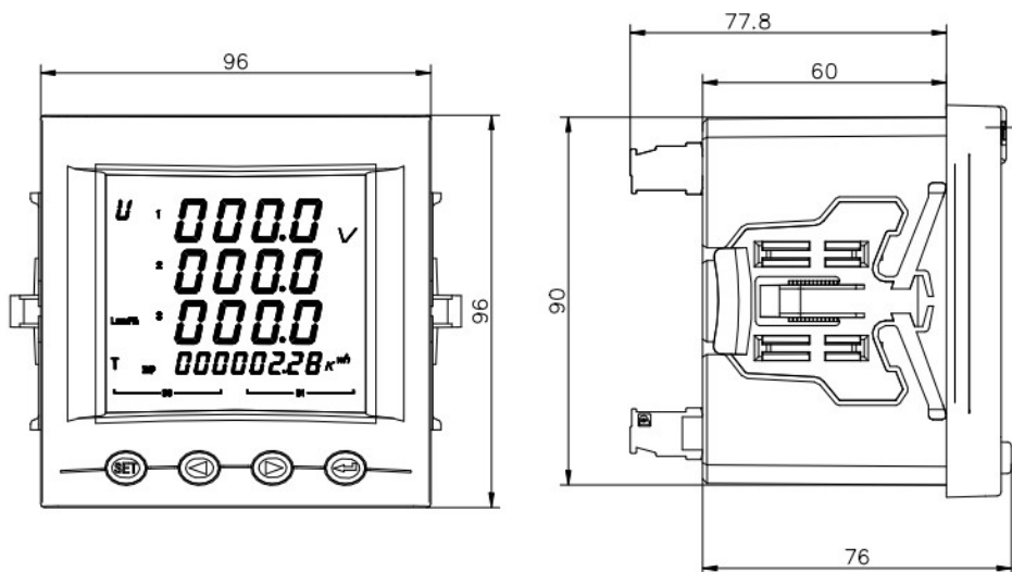
图 2 PM96B 外观尺寸
