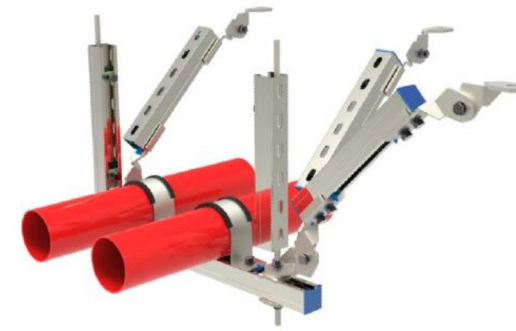
双管多向抗震支架
