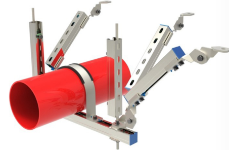
DN200以上单管双向抗震支架
