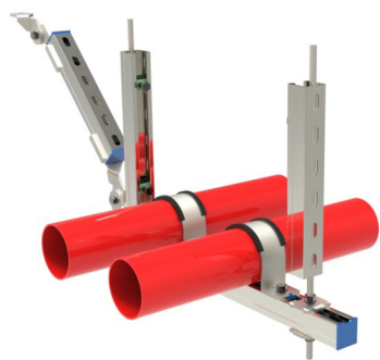
多管侧向抗震支架
