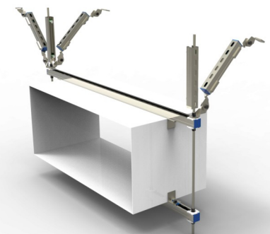
矩形风管双向抗震支架
