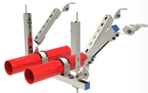
多管双向抗震支架
