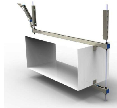
矩形风管侧向抗震支架
