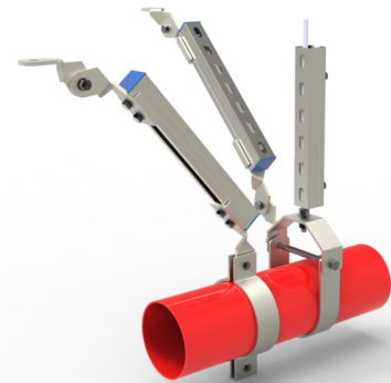
DN200以下单管双向抗震支架
