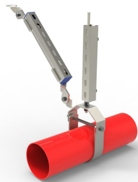
DN200以下单管侧向抗震支架
