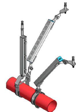
单管侧纵向抗震支架
