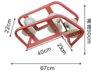
井口大弯 (好尼龙轮)
