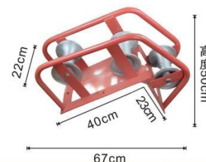
井口大弯 (铝轮)
