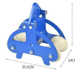
吊架两轮好尼龙轮 重: 10公斤
