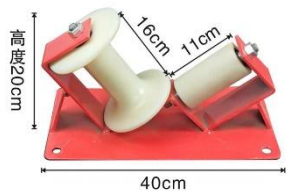
两轮转角 (好尼龙轮) 重量:7KG
