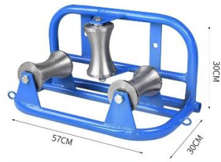
重型转角钢轮 重: 19公斤
