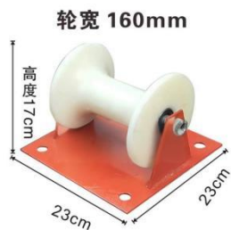
平板滑轮 (好尼龙轮)
