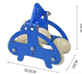
吊架小三轮好尼龙轮 重: 10.6公斤
