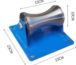
加厚平板不锈钢轮 重: 6.6公斤
