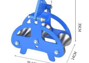
重型吊架小三轮钢轮 重: 17公斤
